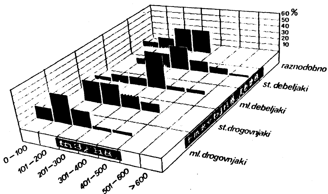
Slika 5: Frekvenčna porazdelitev ocen lesne zaloge (delež vzorcev z določeno lesno zalogo) po posameznih stratumih
